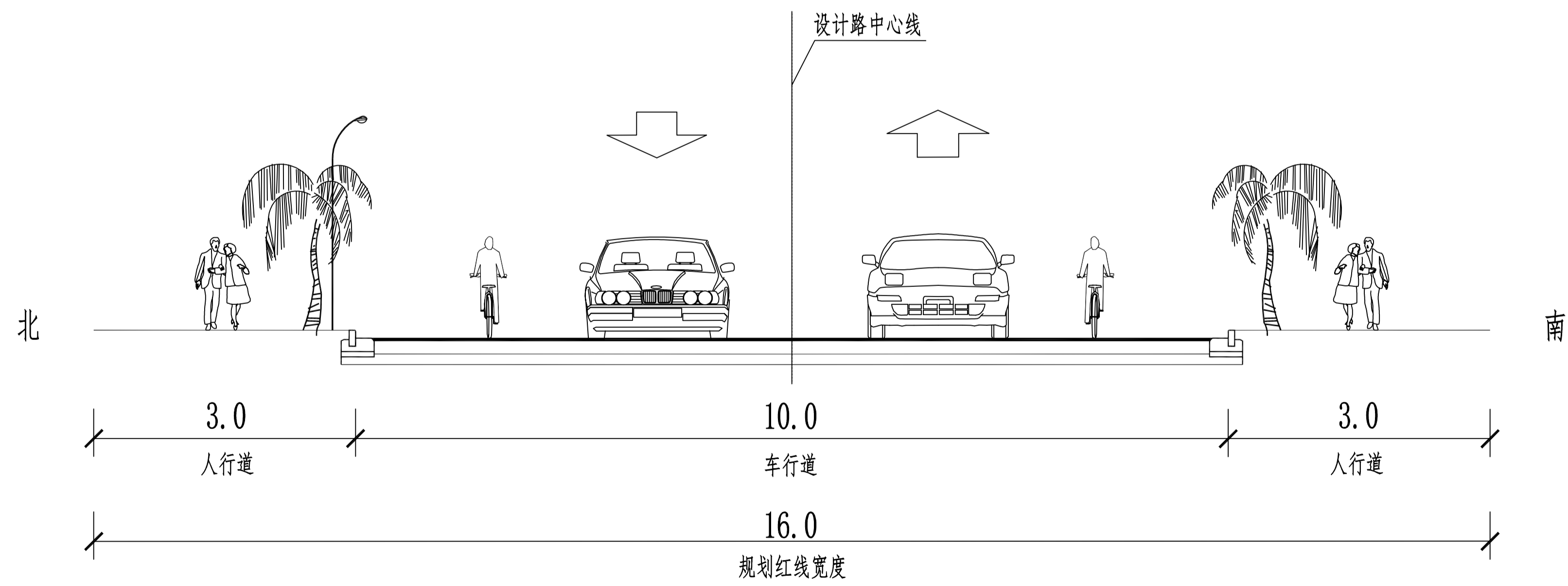
标准横断面设计图
