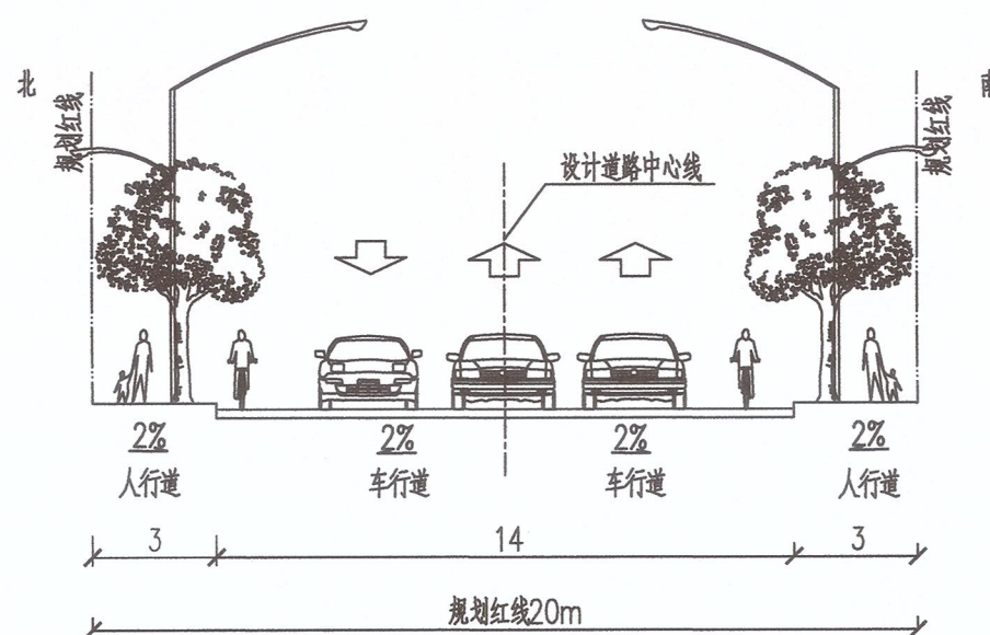
礼泉路与静宁路交叉口横断面
