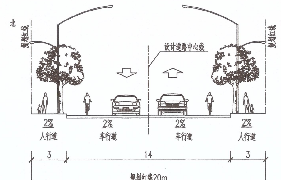
礼泉路道路标准横断面
