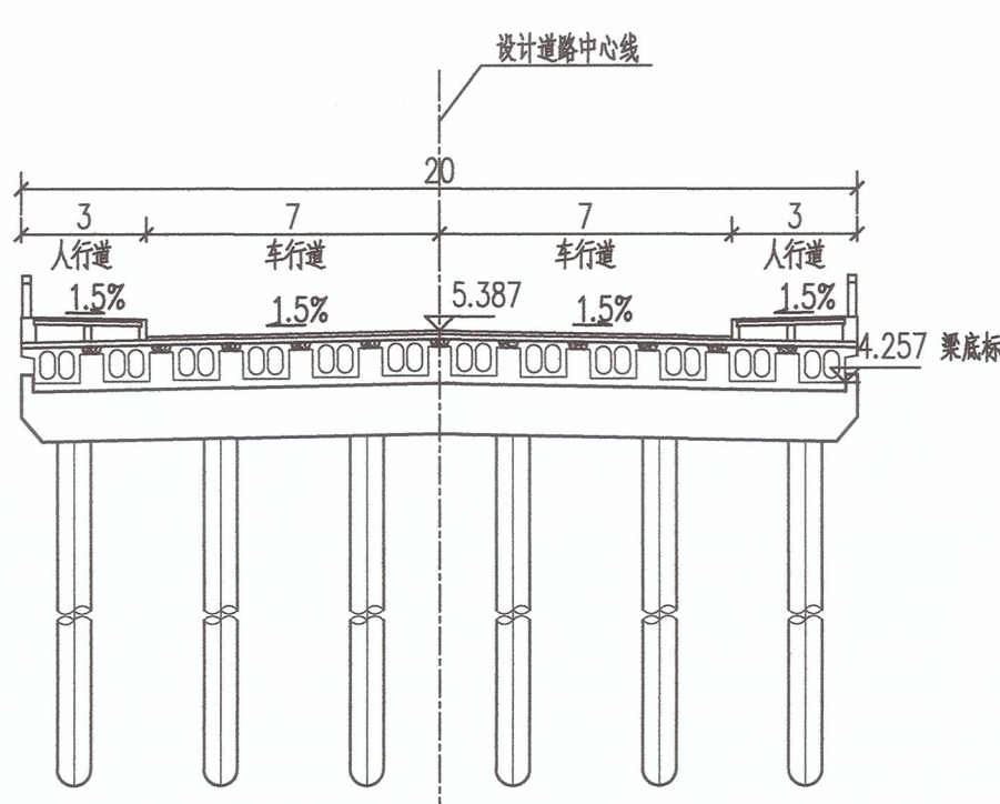
桥墩断面
