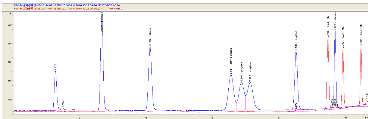
图B.1 苯、甲苯、乙苯、对一二甲苯、间一二甲苯、邻一二甲苯、1,3,5—三甲苯、苯乙烯、1,2,4—三甲苯和1,2,3—三甲苯色谱图
